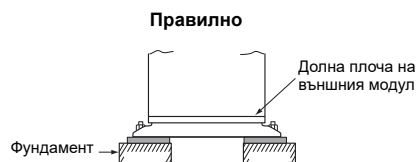
Поддържане на дънната повърхност върху фиксиращия крак, който е в контакт с дъното на външното тяло.
