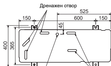
Монтажен отвор на отводнителната дюза Дренажен отвор
