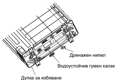
Дренажен нипел
